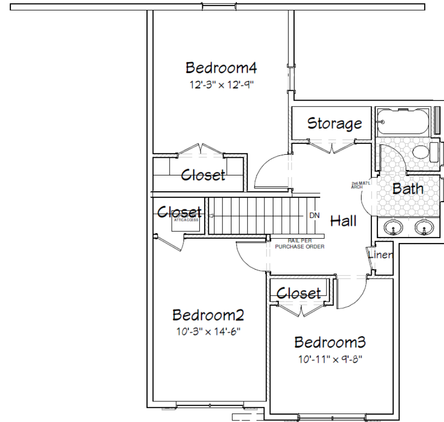
Optional Plan Upper Level
